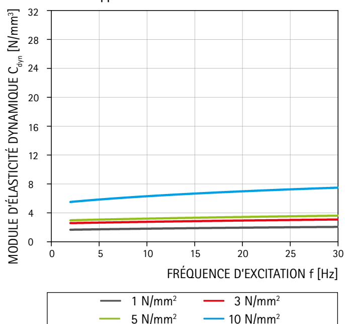
Dimensions de l'appui : 200 x 200 mm
