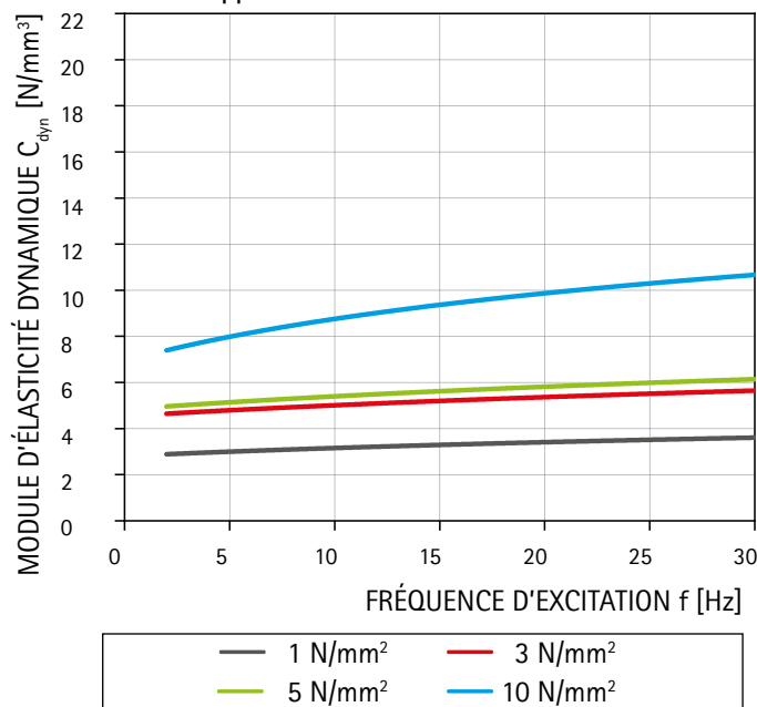
Dimensions de l'appui : 240 x 240 mm
