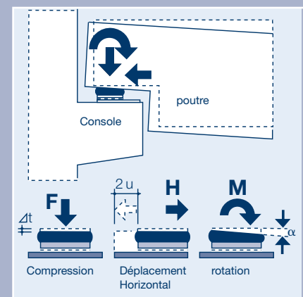
Figure 2. Fonctions des appuis Ciparall®
