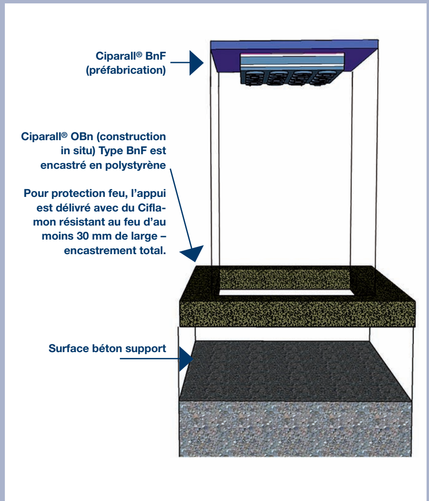
Figure 10. Principe d'installation CIPARALL® type BnF ou OBn sur un poteau
